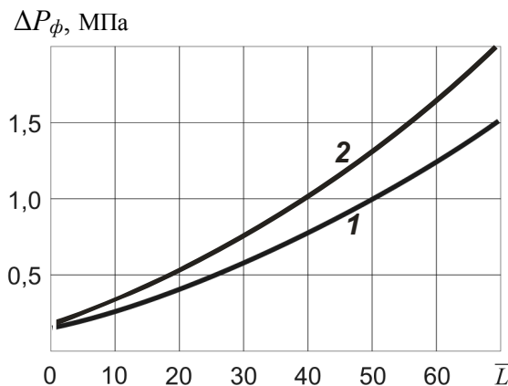
Рис. 1. Зависимость избыточного давления в зоне взрыва от безразмерной длины выработки: 1 – при взрыве метана; 2 – при взрыве метана и угольной пыли
